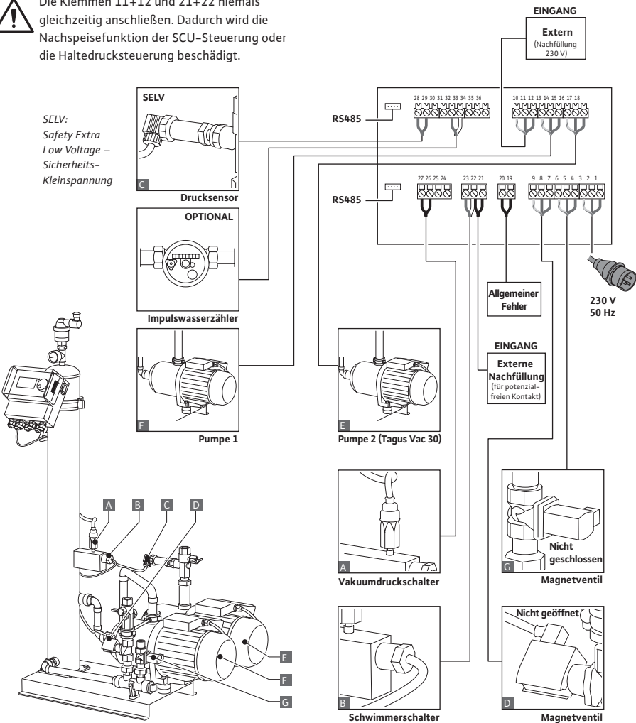
Schwimmerschalter
